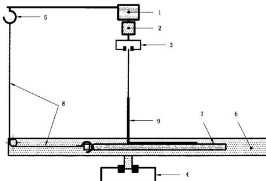
a) 试验装置示意图
